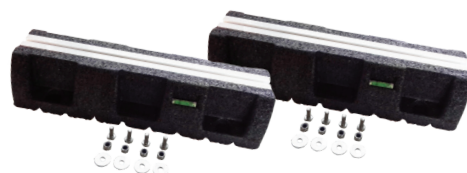
BASE ANTIVIBRANTE A PAVIMENTO IN GOMMA VULCANIZZATA (ALTEZZA DA TERRA MM 95) CON LIVELLA E VITERIE PER BOOSTER HR 3.0 - 7.8
